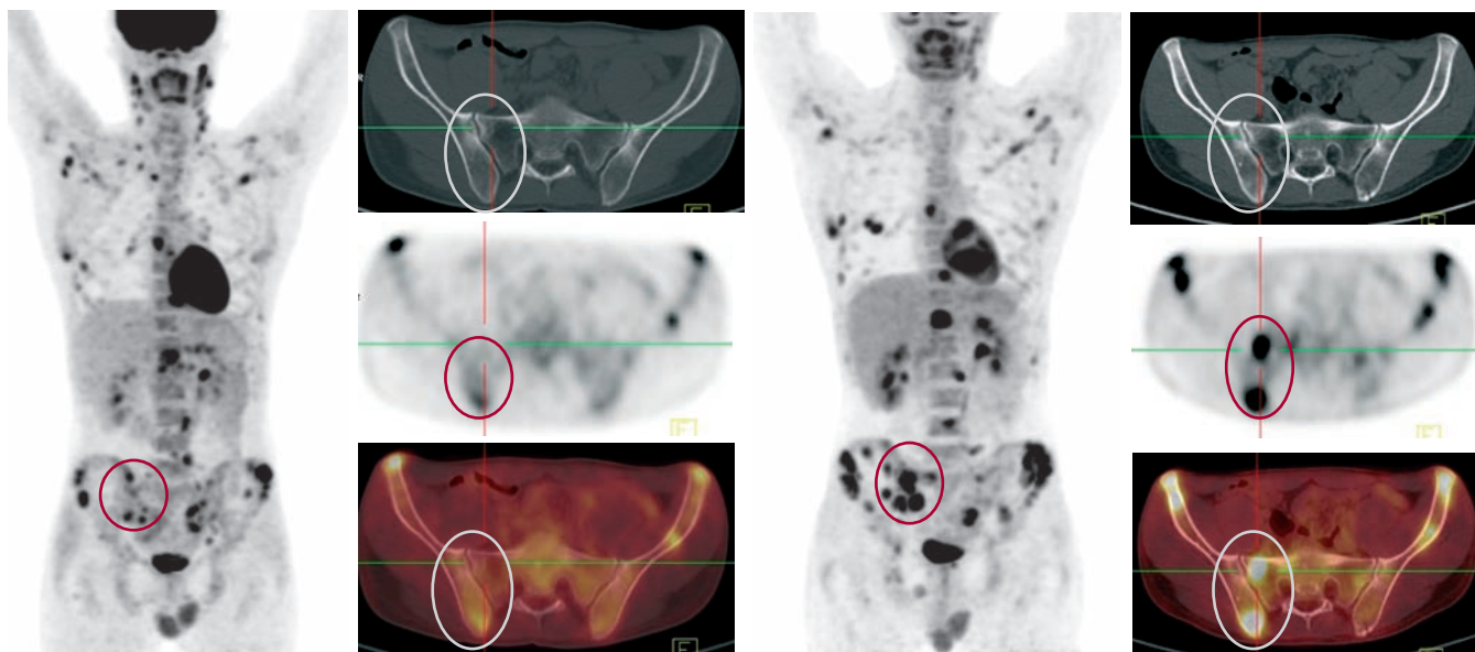
Рис. 10. Оценка эффективности лечения по результатам ПЭТ. У больного с повторным рецидивом лимфомы Ходжкина результаты ПЭТ, выполненной до начала лечения, подтвердили поражение периферических, забрюшинных и подвздошных лимфатических узлов, а также повторное множественное очаговое поражение костного мозга. По результатам КТ в костном мозге костей таза определялись нечеткие участки «замелованности», обусловленные склеротическими процессами в местах его предшествующего поражения (ПЭТ-положительные и сомнительные КТ-отрицательные данные). После 4 циклов противорецидивного лечения результаты ПЭТ свидетельствовали о прогрессировании заболевания (5 баллов по шкале Deauville). При частичной резорбции опухоли в лимфатических узлах выявлено нарастание метаболической активности специфической ткани в определяемых ранее очагах в костном мозге и появление новых. По результатам КТ эффект лечения был расценен как положительный за счет уменьшения размеров лимфатических узлов, тогда как отрицательная динамика процесса в костном мозге по результатам КТ оценена быть не могла и осталась нераспознанной (ПЭТ-положительные и КТ-отрицательные данные)
