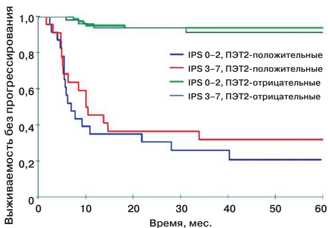
Рис. 5. Выживаемость без прогрессирования больных с распространенными стадиями лимфомы Ходжкина согласно международному прогностическому индексу (IPS) и результатам промежуточной ПЭТ после 2-го цикла полихимиотерапии [37]. Результаты промежуточной ПЭТ позволили с высокой точностью идентифицировать больных с хорошим прогнозом (ПЭТ-отрицательных, у которых 3-летняя выживаемость без прогрессирования составила 95 %) и прогностически неблагоприятных (ПЭТ-позитивных, у которых 3-летняя выживаемость без прогрессирования составила 28 %)
