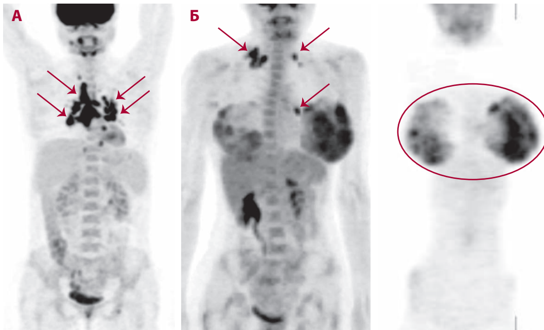
Рис. 2. Позитронно-эмиссионная томография. Активное накопление ^{18}\text{F} -ФДГ:
