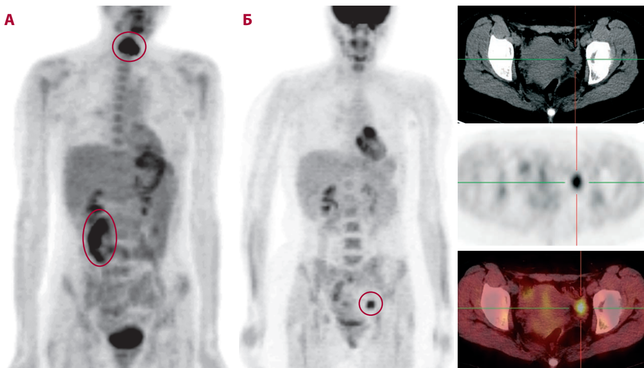
Рис. 1. Позитронно-эмиссионная томография. Активное накопление ^{18}\text{F} -ФДГ: А — в голосовых связках и спазмированном кишечнике; Б — в физиологически активном яичнике
