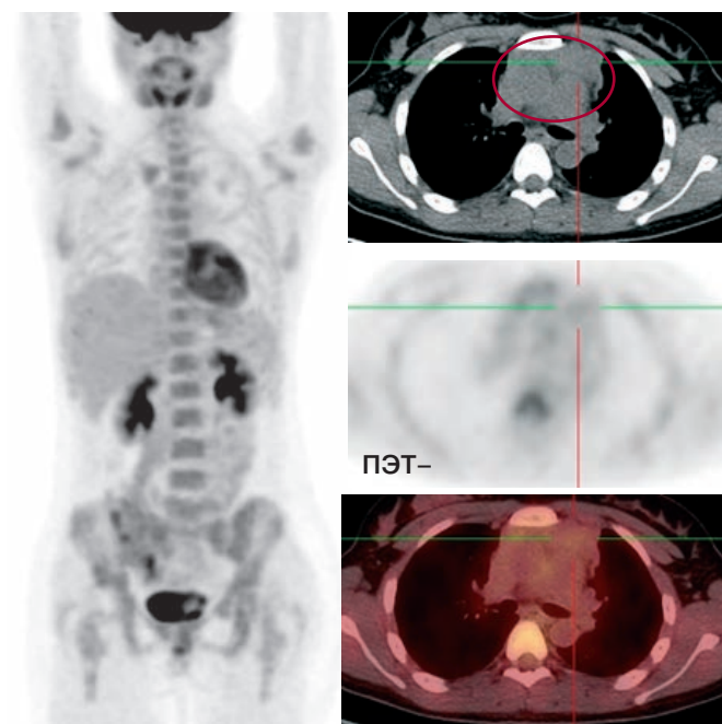
Рис. 7. Пример оценки эффективности лечения по результатам ПЭТ. У больного лимфомой Ходжкина данные ПЭТ до лечения подтвердили II стадию заболевания с массивным поражением средостения (поперечный диаметр опухоли 84 мм). После 2 циклов полихимиотерапии: по КТ определялось существенное уменьшение опухоли (до 40 мм в поперечном диаметре); результаты ПЭТ оценены в 2 балла по шкале Deauville, что свидетельствовало о полном метаболическом ответе на лечение и благоприятном прогнозе, т. е. метаболическая активность резидуальной массы не превышала уровень метаболизма в других отделах средостения. Для больных, включенных в клинические исследования, подобный результат (1 или 2 балла) подразумевает возможность деэскалации первоначально запланированного лечения. Получение аналогичных данных ПЭТ после завершения лечения (химио- или химиолучевой терапии) подтверждает полную ремиссию
